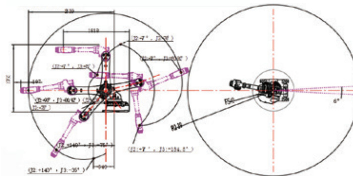
机械手法兰连接图 Robot Flange Connection Diagram
