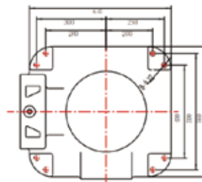
机械手底座安装图 Robot Base Installation Diagram
